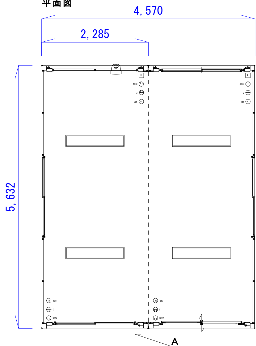
平面図
