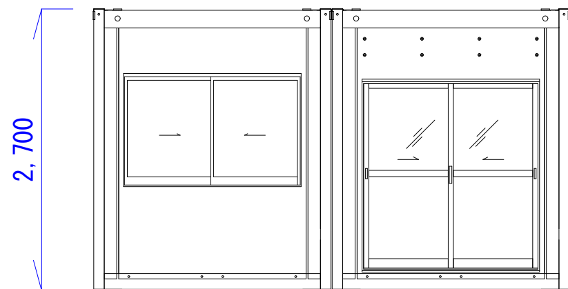
A 立面図
