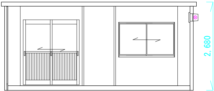
A 立面図
