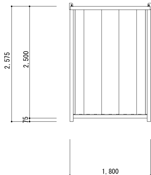
D面 立面図 S=1/50
