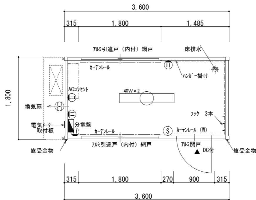
平面図 S=1/50
