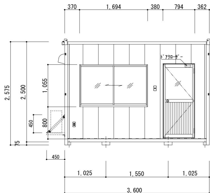
A面 立面図 S=1/50
