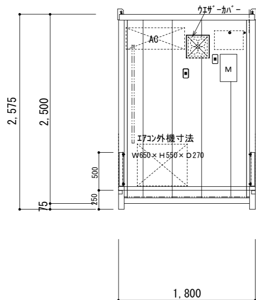
B面 立面図 S=1/50
