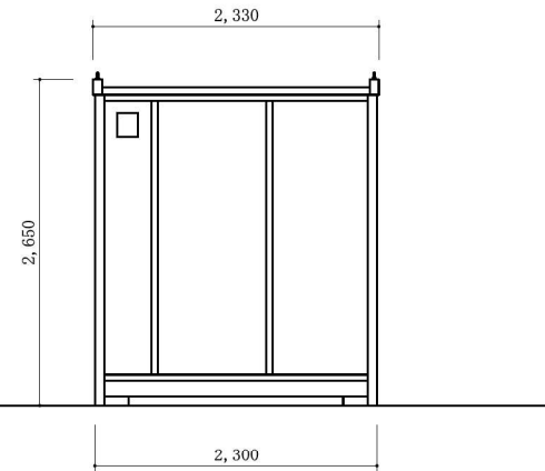
B面立面図
